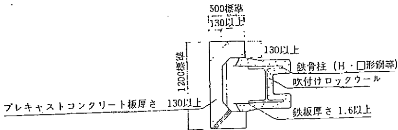
ヨコ目地部詳細図
