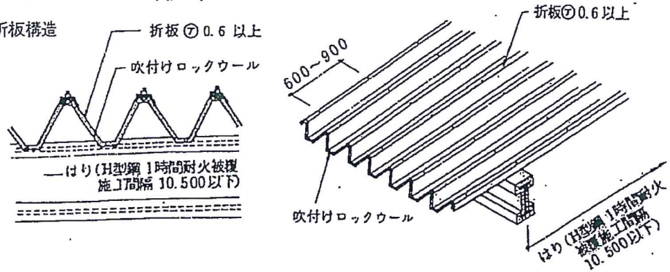
(ロ) 瓦棒構造
