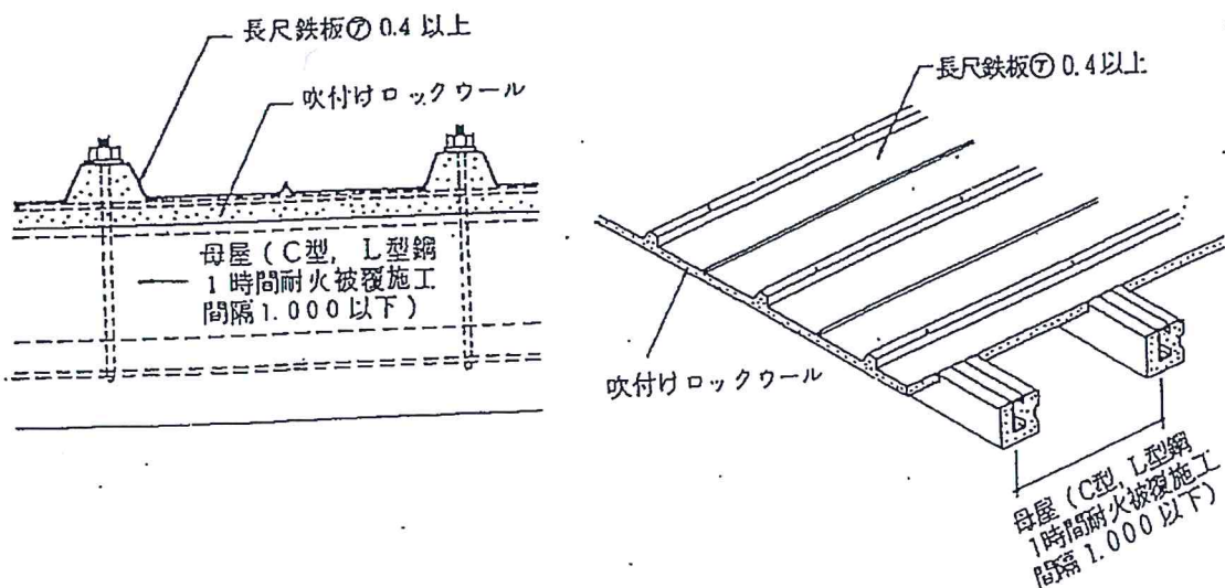
(ハ) 長尺鉄板構造
